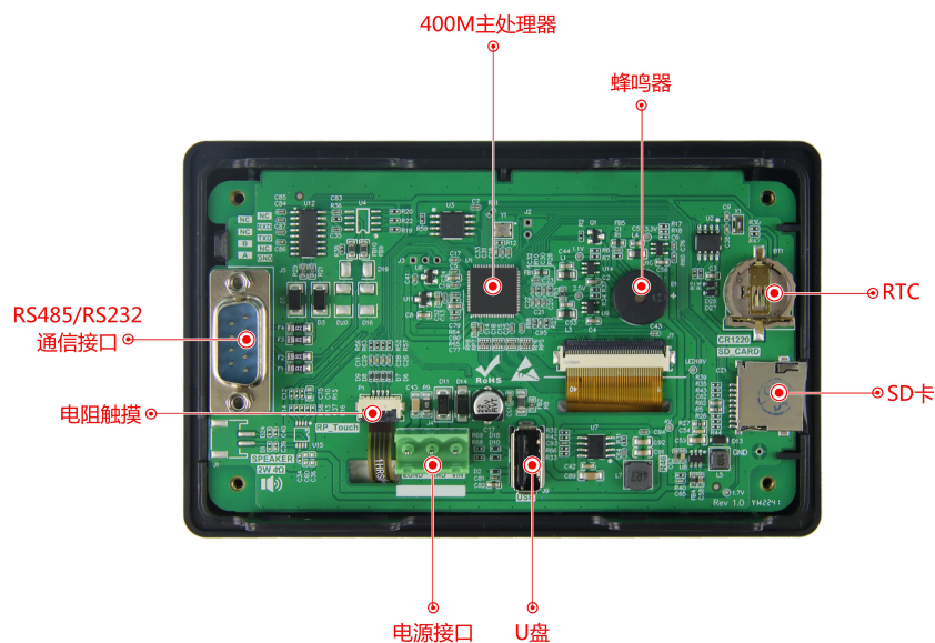
图 1-2 硬件配置图
