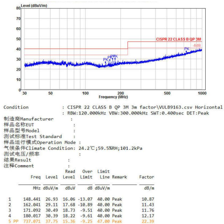
图 7-7 辐射测试垂直方向
