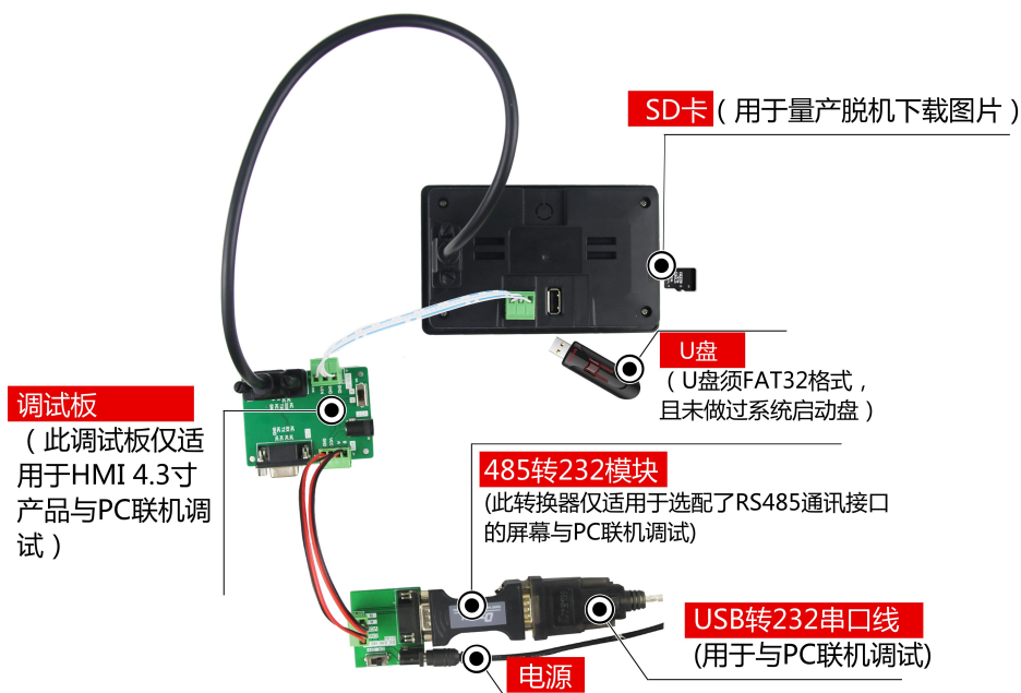
图 1-3 RS485 调试图
