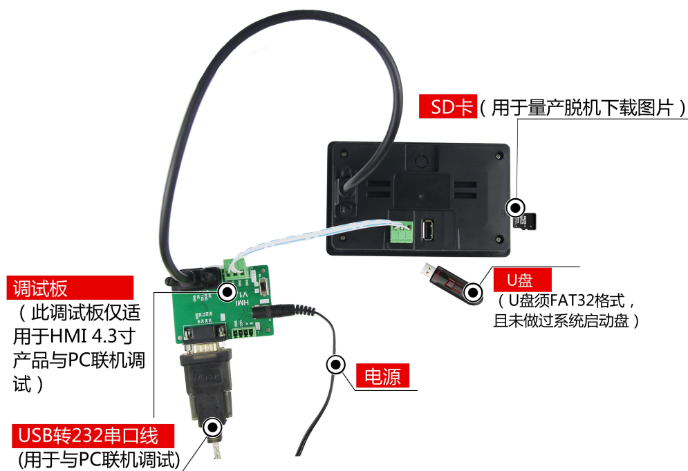
图 1-4 RS232 调试图
