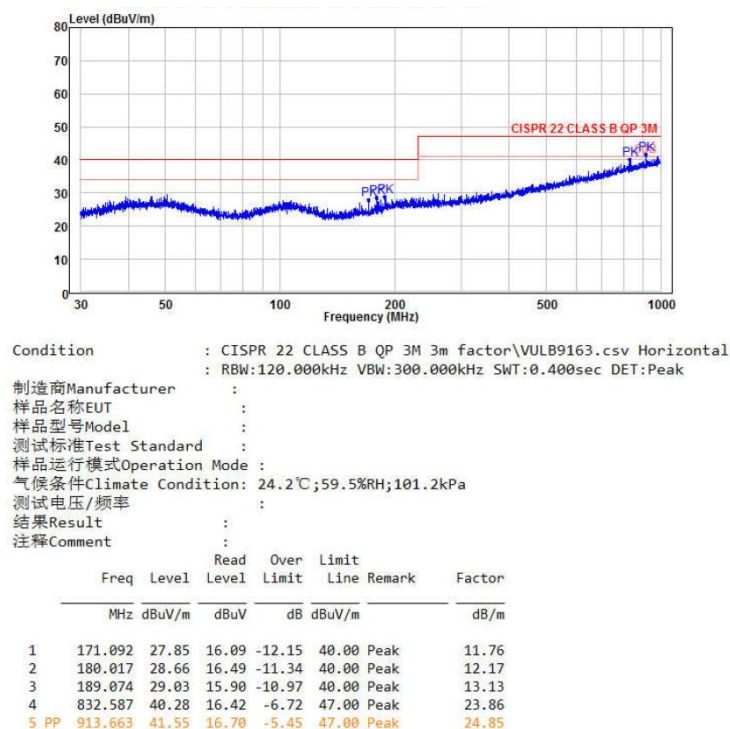
图 7-6 辐射测试水平方向
