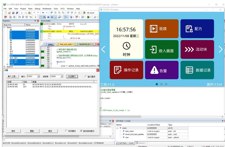
图 12-3Keil 开发环境与虚拟 HMI 绑定调试
